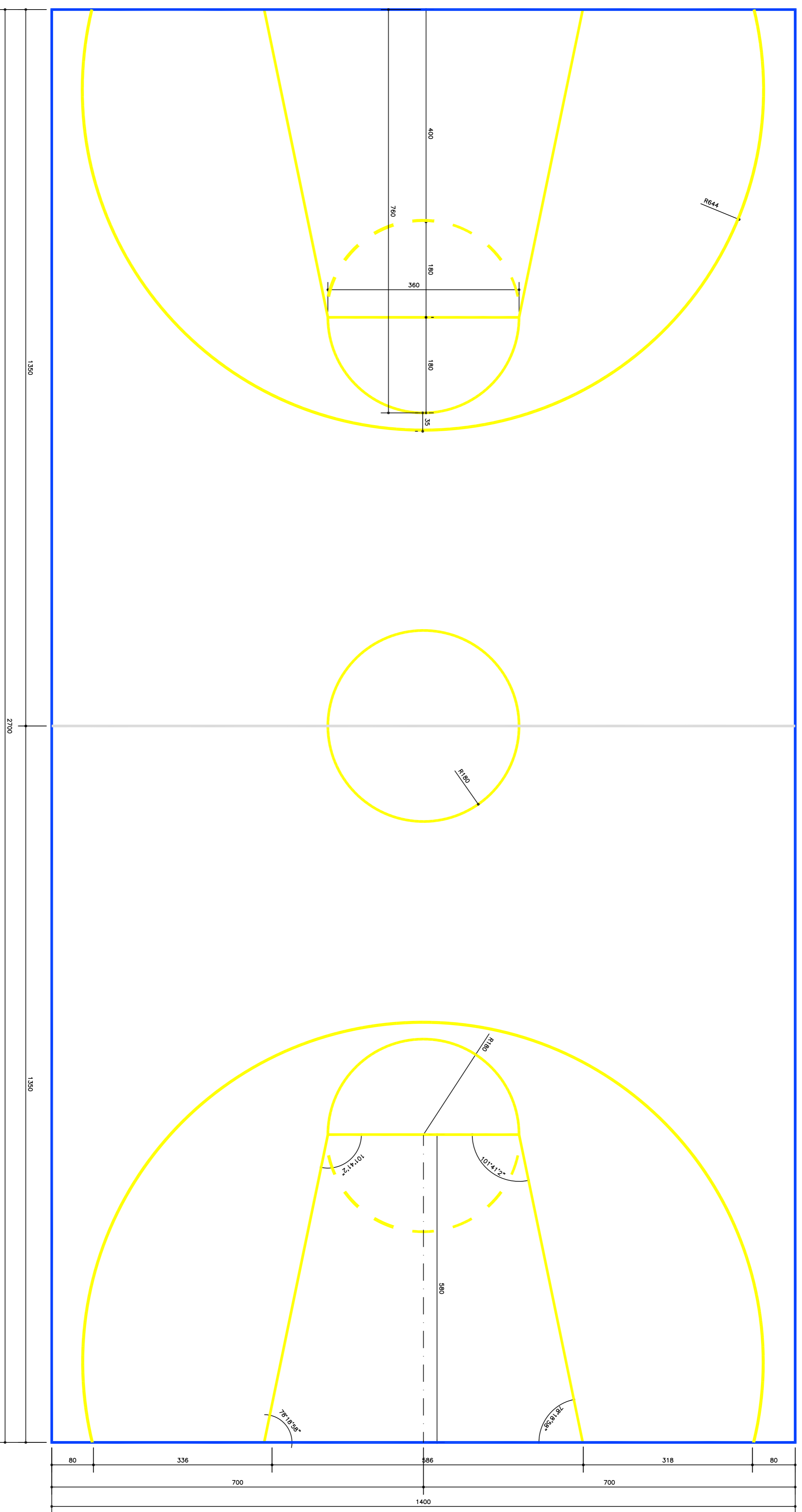
DEMARCAÇÃO DA QUADRA DE BASQUETE FOMM BASQUETE COM AMPLIAÇÃO ESCALA: 1:50 (desenvolvido = sem)
